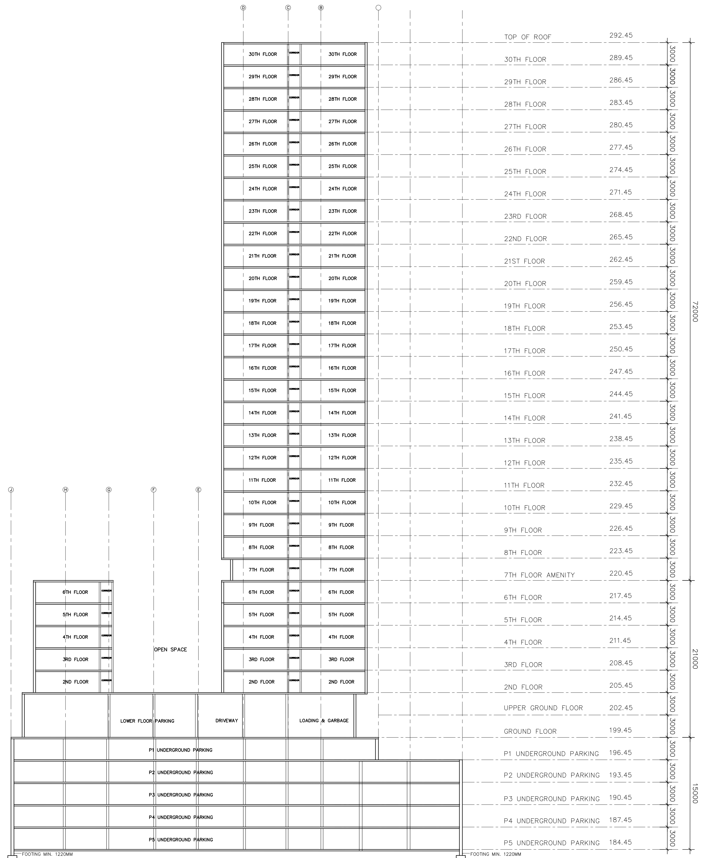
SECTION B-B SCALE: 1:250
