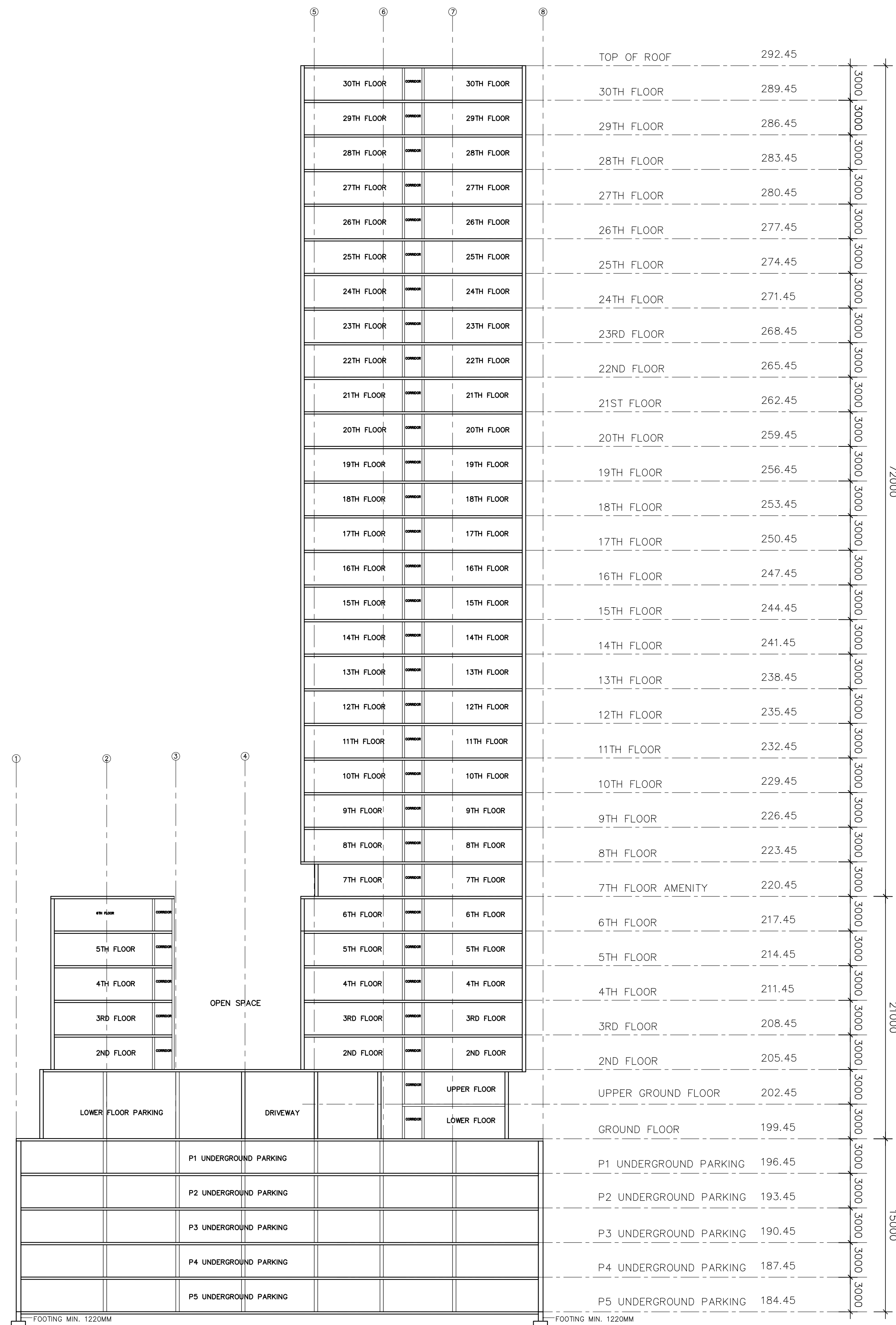
SECTION A-A SCALE: 1:250
